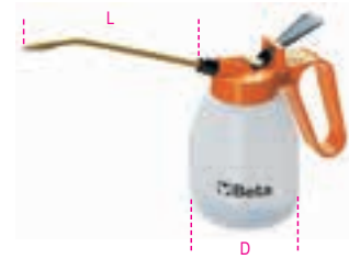
cc D mm L mm 200 67 140 4 017520002 300 77 140 4 017520003 500 95 140 4 017520005 700 95 140 2 017520007
